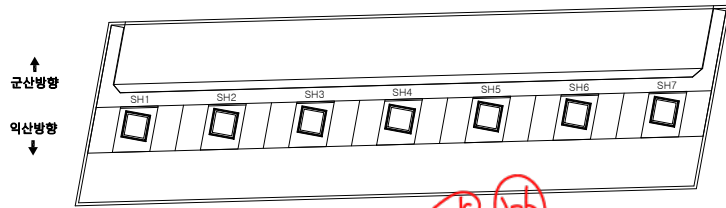
받침상면
